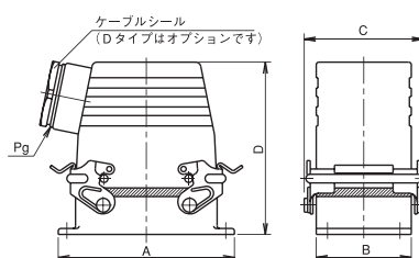
2ロックレバー式
