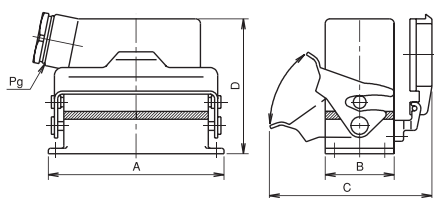
1ロックレバー式 カバー付
